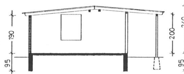
SCHNITT A - B
