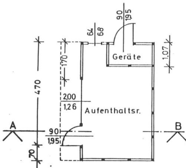
GRUNDRISS
