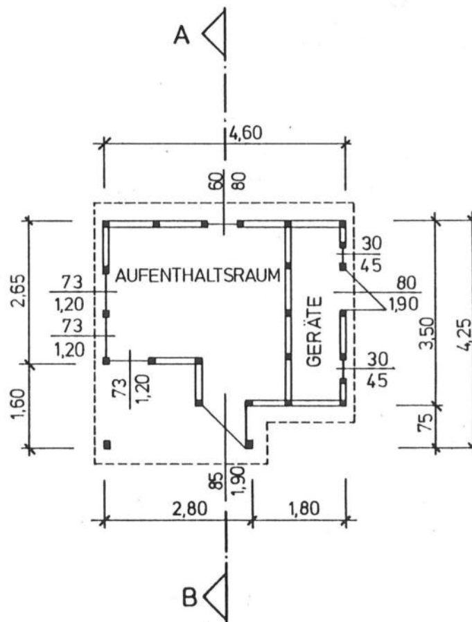
GRUNDRISS
