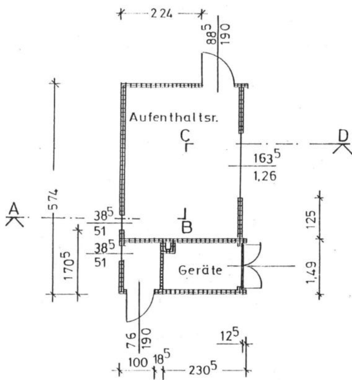
GRUNDRISS
