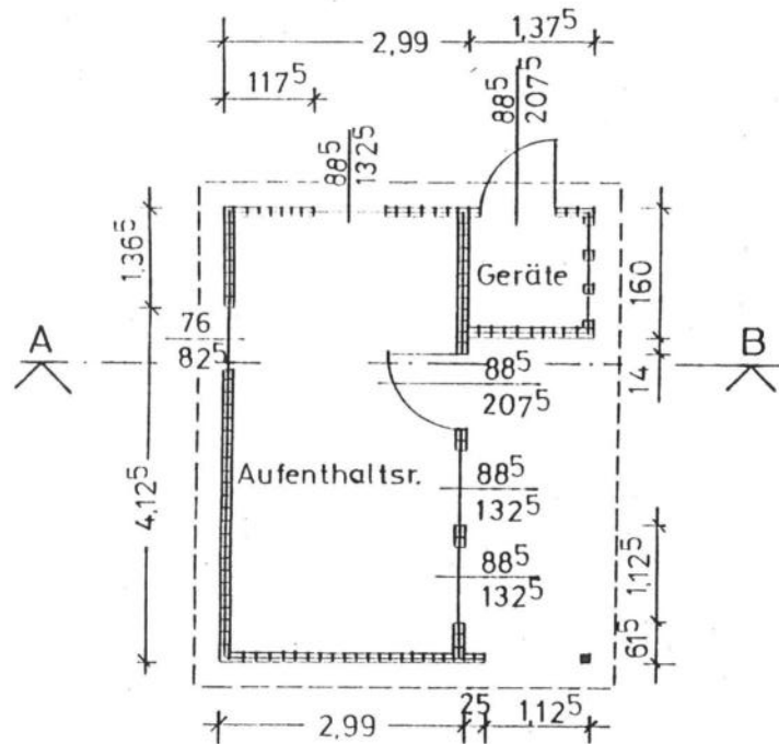
GRUNDRISS
