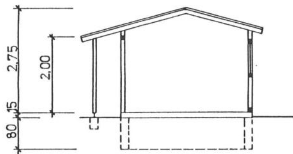
SCHNITT A - B
