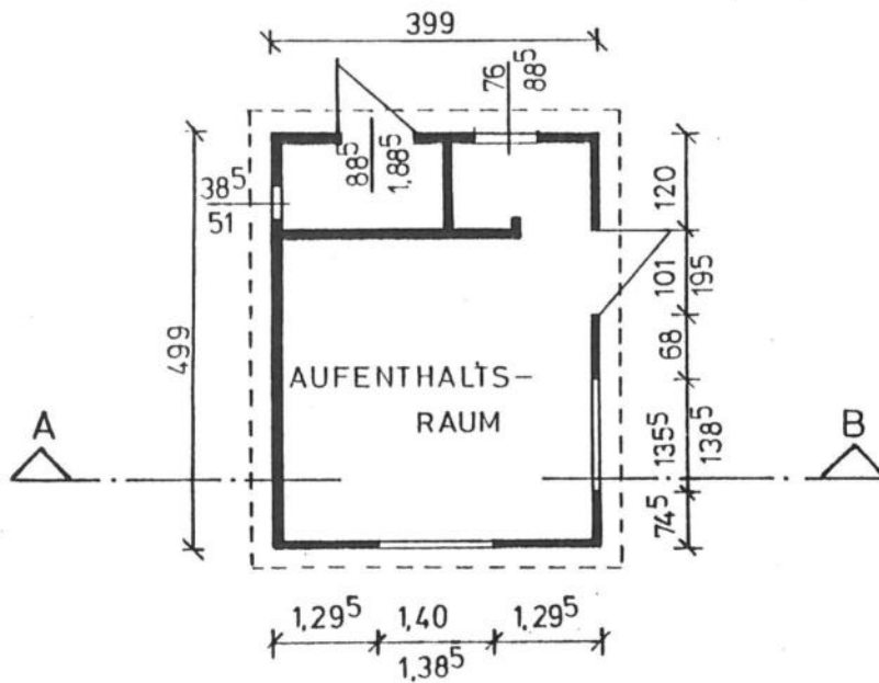
GRUNDRISS
