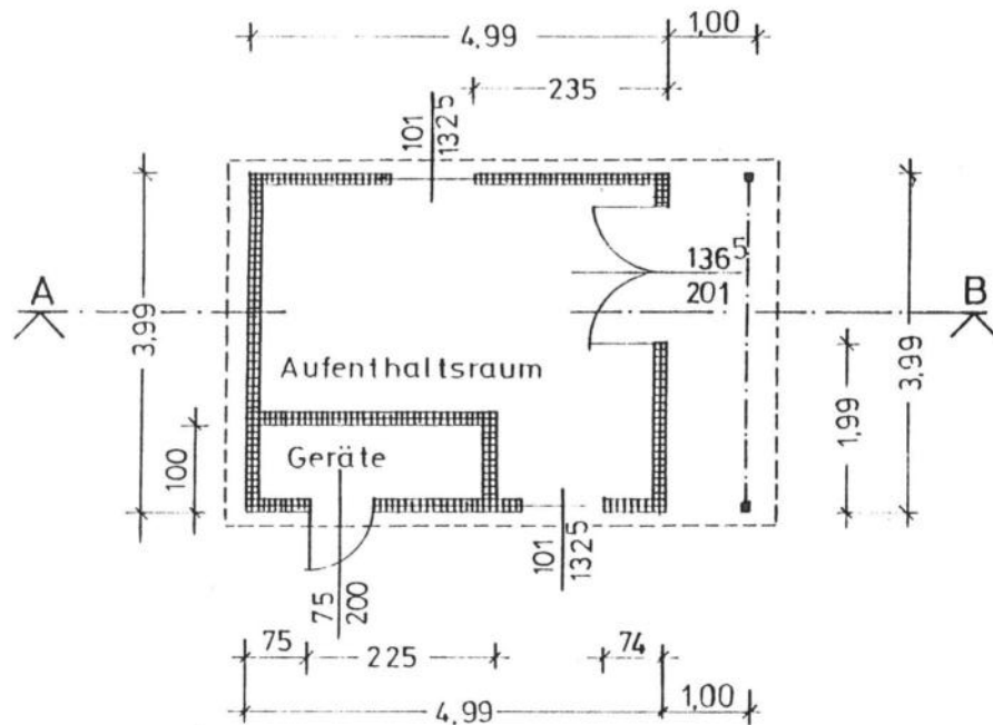
GRUNDRISS
