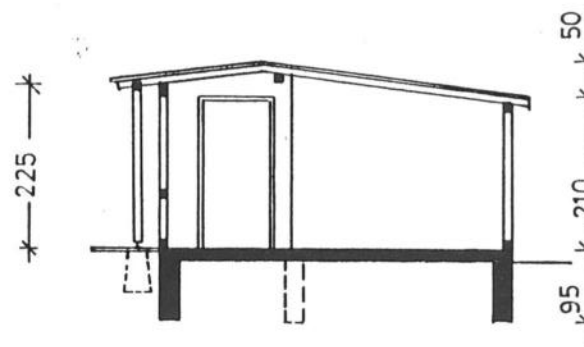
SCHNITT A - B
