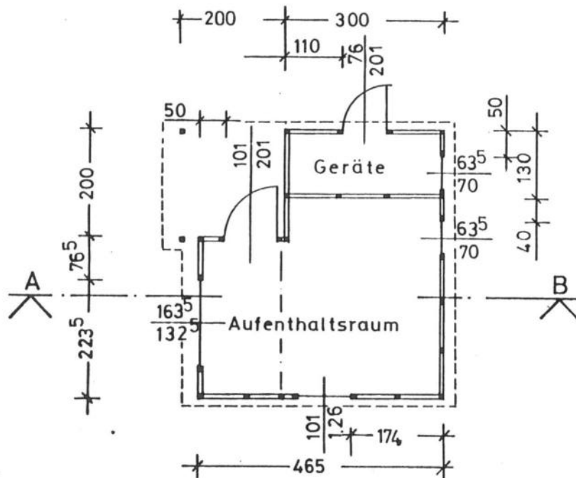
GRUNDRISS
