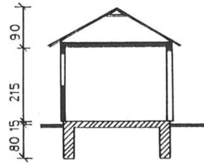
SCHNITTA - B
