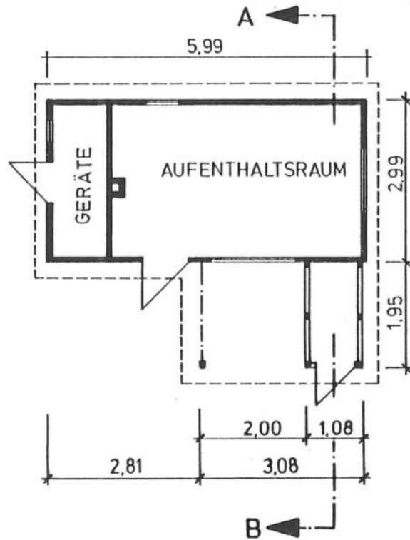
GRUNDRISS
