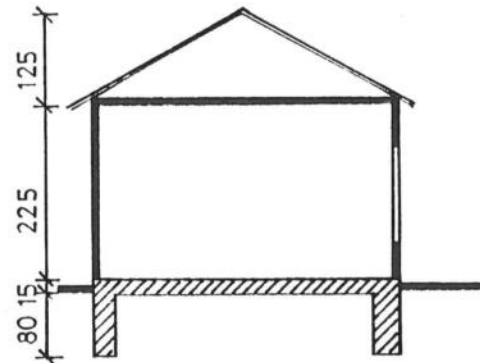
SCHNITT A-B
