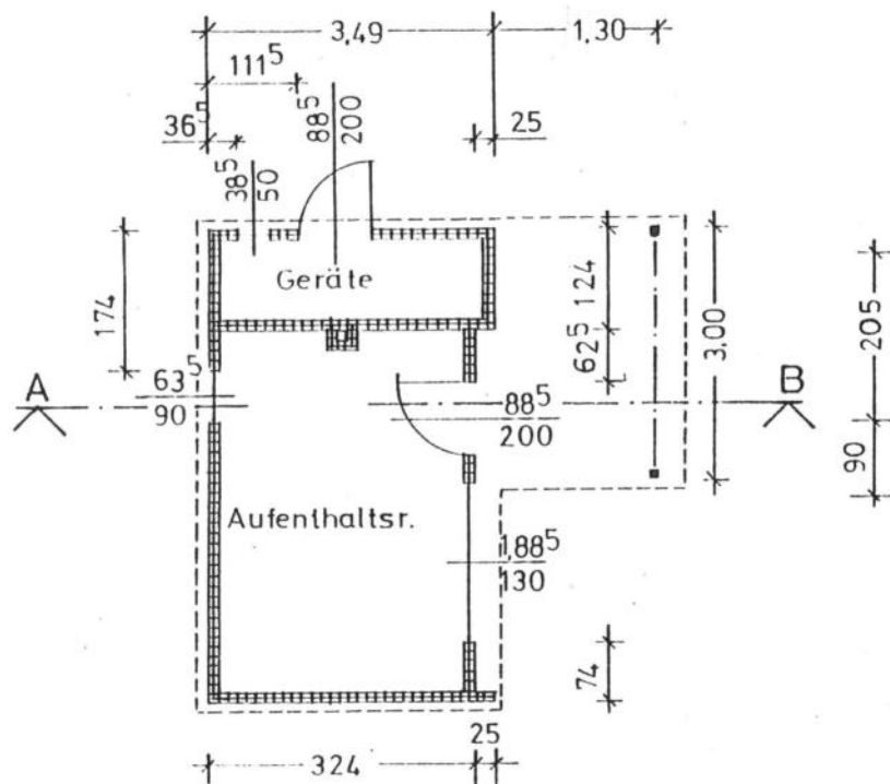
GRUNDRISS
