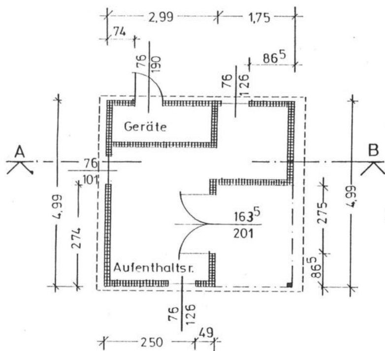
GRUNDRISS
