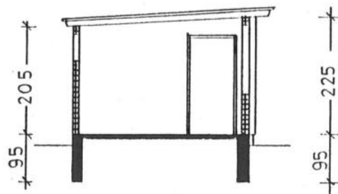
SCHNITT A - D
