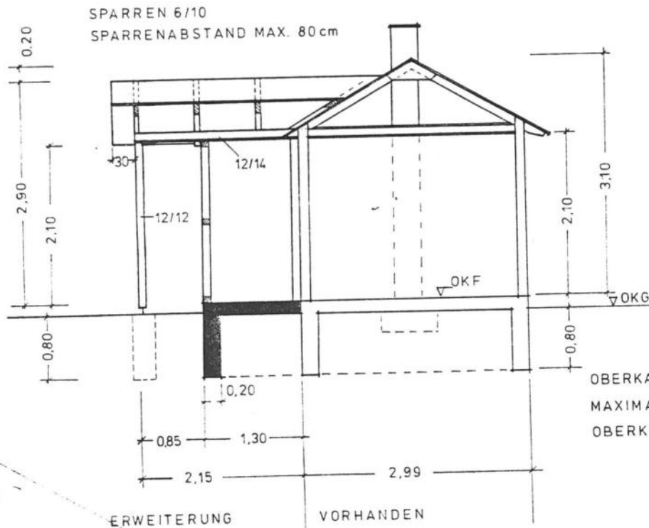
SNITT B - A
